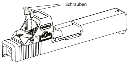
Abb. 5 Montage auf einem Schlitten
